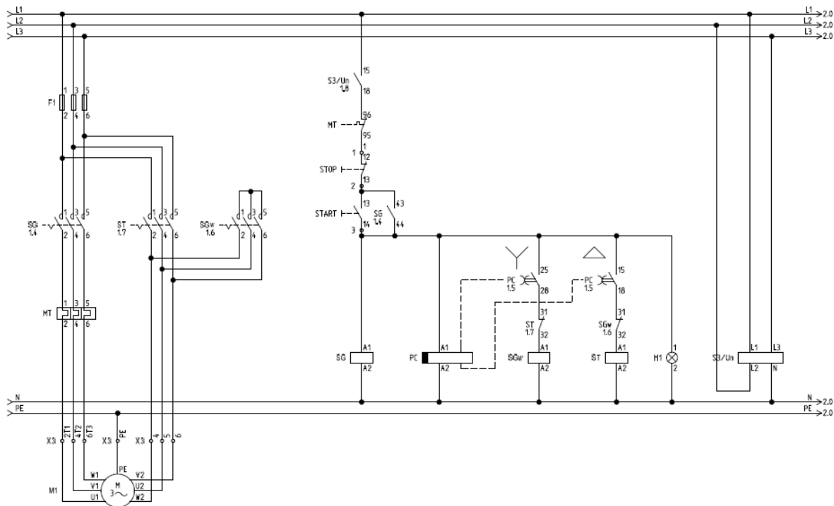
Schemat podstawowy połączeń przełącznika gwiazda trójkąt
